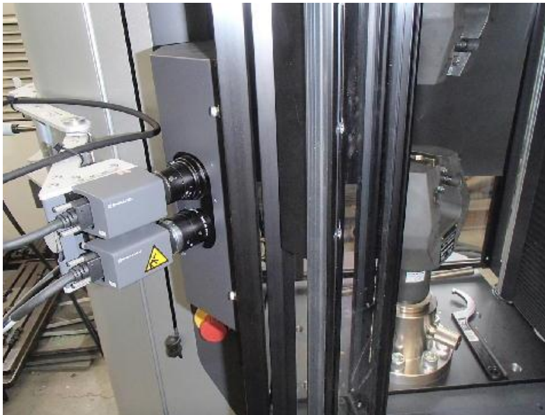
図3 非接触式ビデオ伸び計 (カメラ視野 120ミリメートル及び800ミリメートル ダブルカメラ方式)
