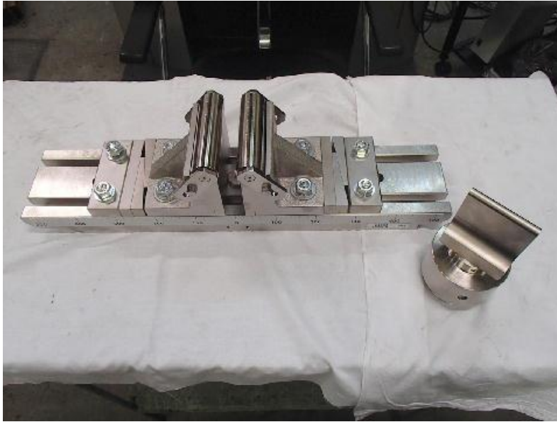
図2 金属用3点曲げ治具 (最大容量 100キロニュートン、支点間距離 最大500ミリメートル)
